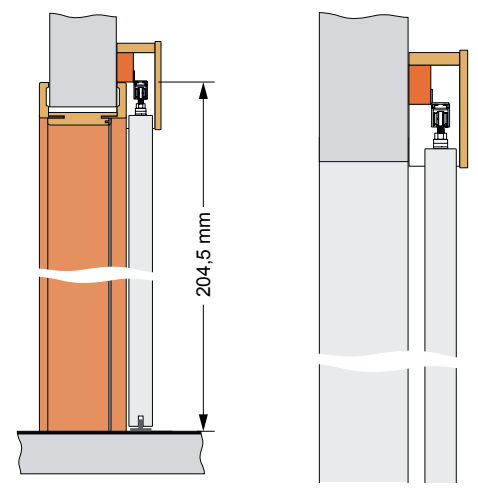
Nástěnný posuvný systém s obložkovou zárubní.
