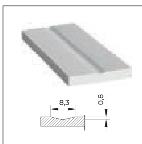
detail frézování
