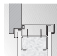
zároveň Rohová VELKÁ montáž na stěně SDK
