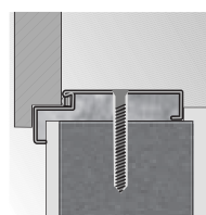
zároveň Rohová VELKÁ montáž pomocí hmoždinek
