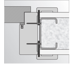
montáž pomocí šroubů do stěny SDK
