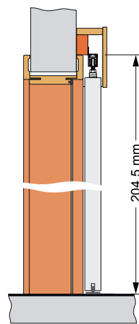
Nástěnný posuvný systém s obložkovou zárubní.
