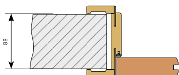
obl. zárubeň B (88-108 mm) síla stěny 90 mm zasunutý zákloповý límeč
