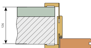
obl. zárubeň B (95-115 mm) síla stěny 126 mm zákloповý límeč s delším spojovacím perem +18 mm
