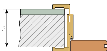
obl. zárubeň B (88-108 mm) síla stěny 110 mm zákloповý límeč vysunutý v rozsahu regulace 0-20 mm na své maximum
